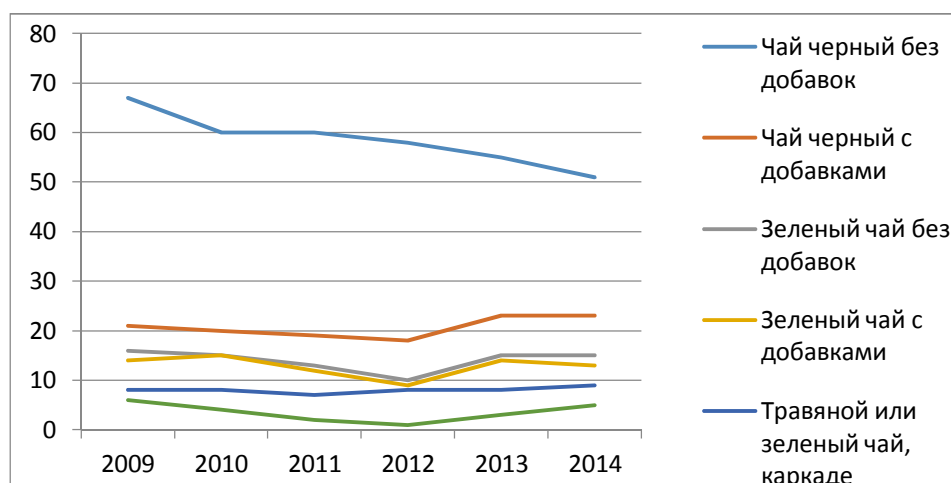
Рис. 3. Лояльность использования видов чаев в течение нескольких лет.
