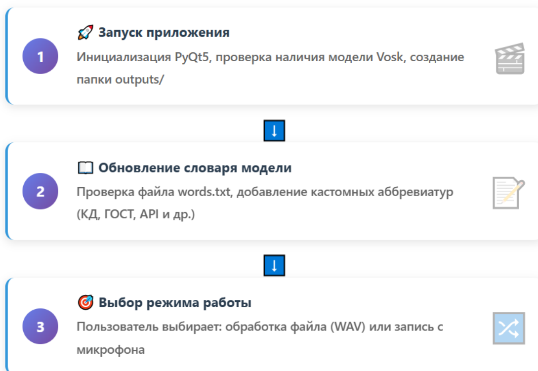
Рис. 2. Алгоритм работы программы
