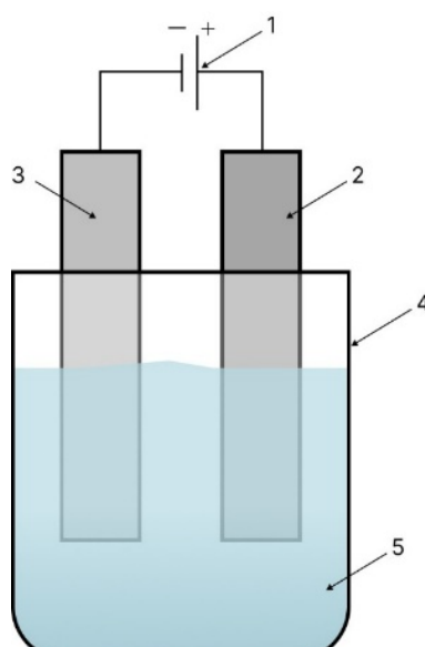
Рис. 1. Схема установки для нанесения цинкового покрытия (1 – источник питания, 2 – стальной анод, 3 – стальной катод, 4 – электролизёр, 5 – электролит)
