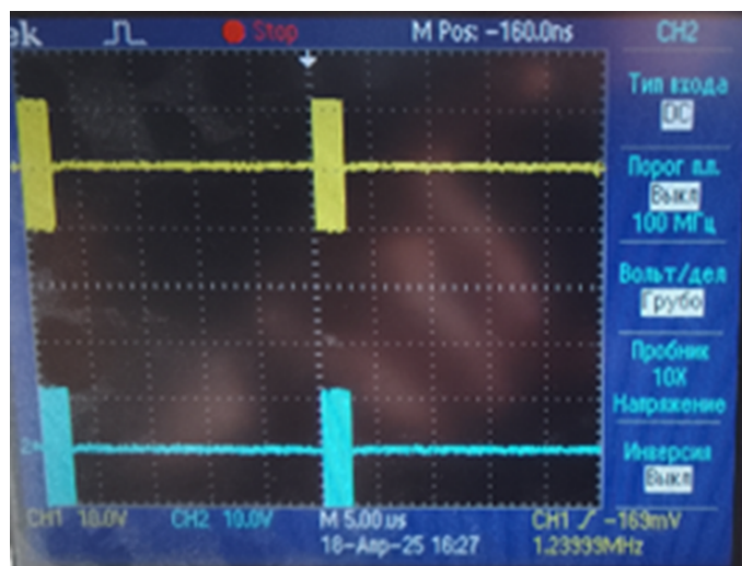
Рис. 3. Формирование радиоимпульса с помощью ЦАП
