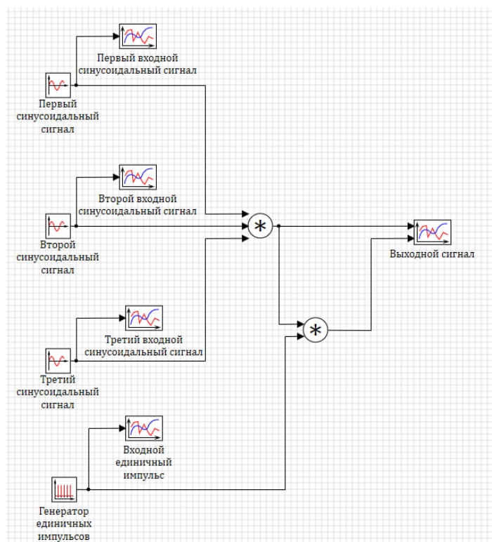
Рис. 4. Схема для формирования дискретного сигнала
