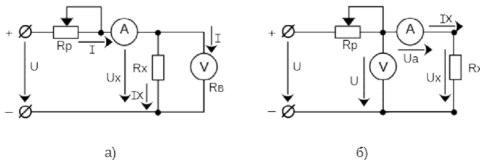
Рис 3 – Схемы включения приборов: а) для малых сопротивлений/больших ёмкостей; б) для больших сопротивлений /малых ёмкостей
