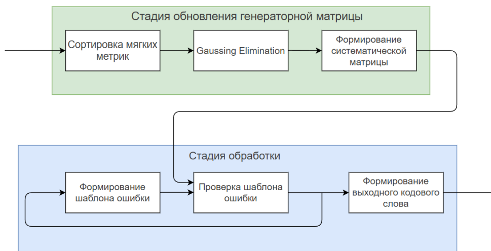
Рис. 1. Структурная схема декодера OSD
