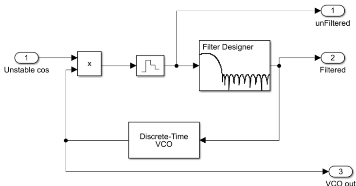
Рис. 4. Подсистема компенсации фазового сдвигов
