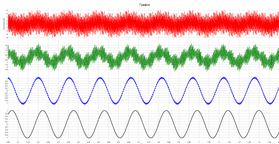
Рис. 2. Временные диаграммы исходного сигнала (красный), сигнала на выходе 1-го каскада (зеленый), на выходе 2-го каскада (синий), 3-го каскада (черный)
