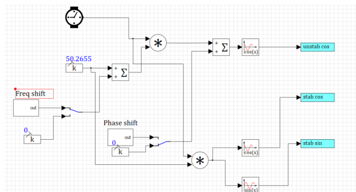
Рис. 8. Подсистема генерации исходного сигнала
