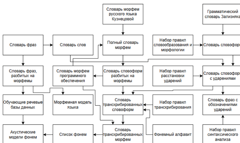
Рис. 3. Базы данных модели SIRIUS для распознавания русской речи
