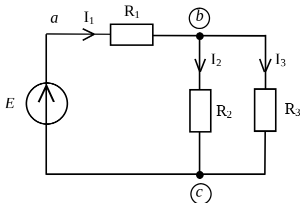
Рис. 1. Схема цепи, исследуемой в лабораторной работе №1
