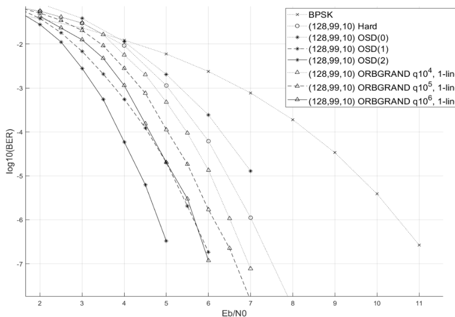
Рис. 4. Результаты моделирования BCH (128,99,10)
