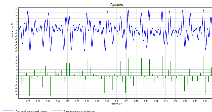
Рис. 6. Выходной аналоговый и дискретный сигналы при частоте дискретизации 615 Гц
