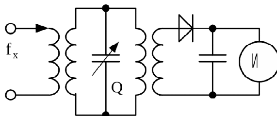
Рис 1. Структурная схема реализации резонансного метода
