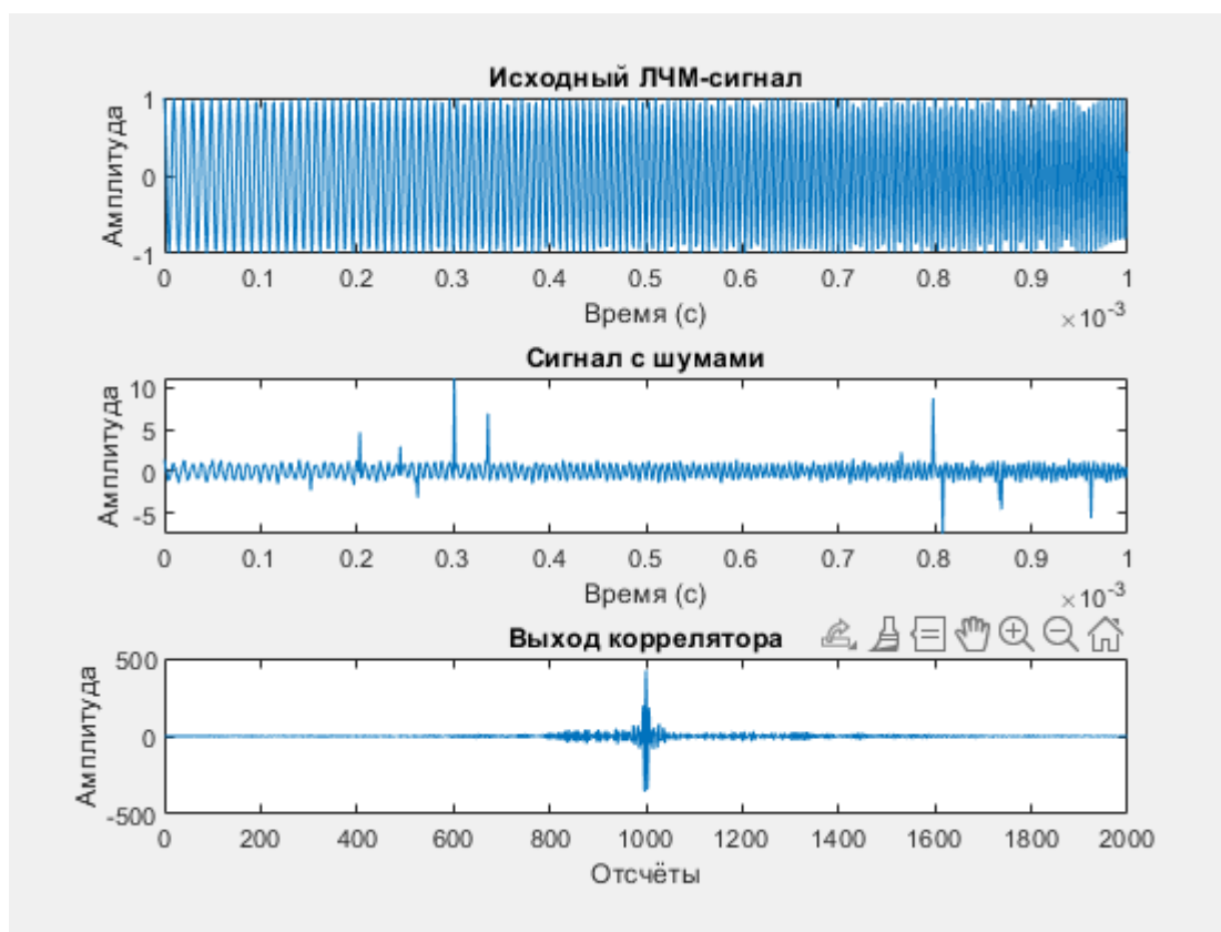
Рис. 2. Результаты моделирования обработки ЛЧМ-сигнала
