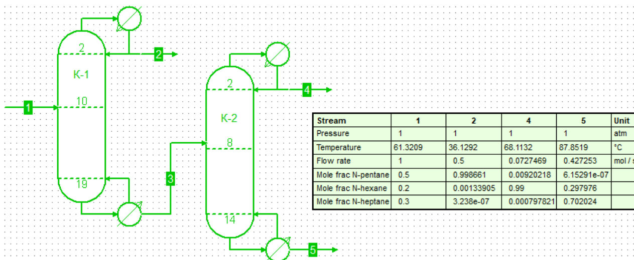
Рис. 5. Рассчитанные программой значение кубового остатка
