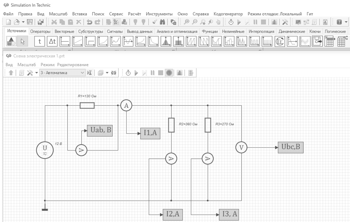
Рис. 2. Имитационная модель исследуемой цепи
