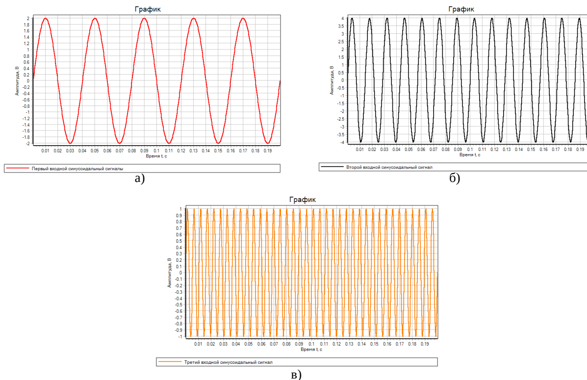
Рис. 2. Сигналы на выходе генератора: а) первый входной синусоидальный сигнал с f_1 = 25 Гц, б) второй входной синусоидальный сигнал с f_2 = 70 Гц, в) третий входной синусоидальный сигнал с f_3 = 190 Гц.
