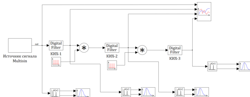
Рис. 1. Модель 3-х ступенчатой структуры узкополосных КИХ-фильтров
