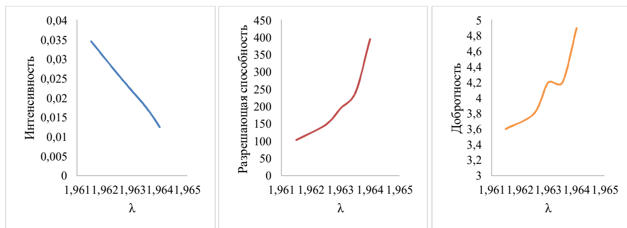
Рис. 2. Зависимости основных качественных характеристик от углового коэффициента при работе с одним квадрупольным масс-фильтром
