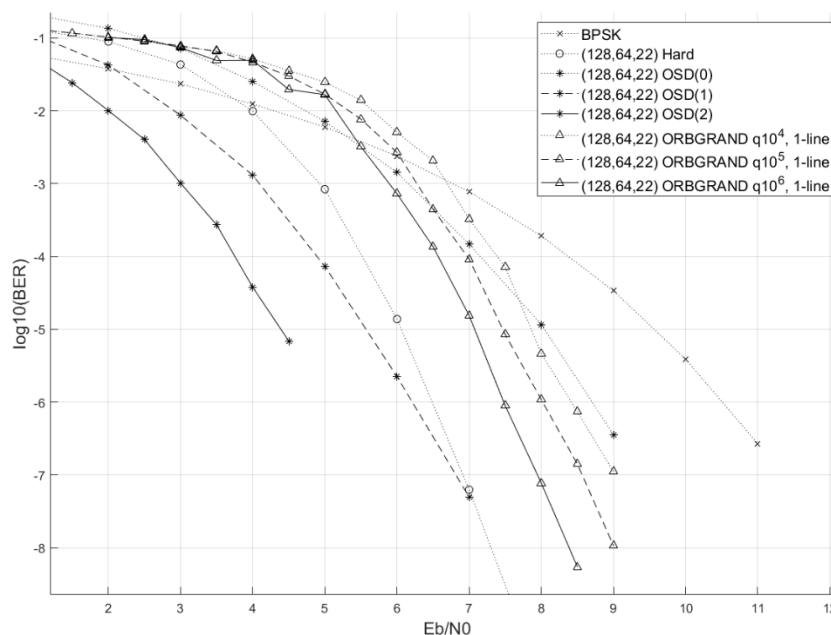
Рис. 3. Результаты моделирования BCH (128,64,22)
