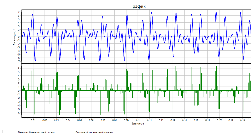
Рис. 7. Выходной аналоговый и дискретный сигналы при частоте дискретизации 1230 Гц
