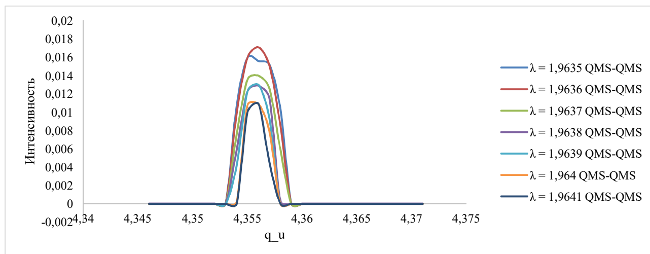
Рис. 3. Влияние углового коэффициента на форму и высоту массовых пиков при работе с тандемом из двух квадрупольных масс-фильтров
