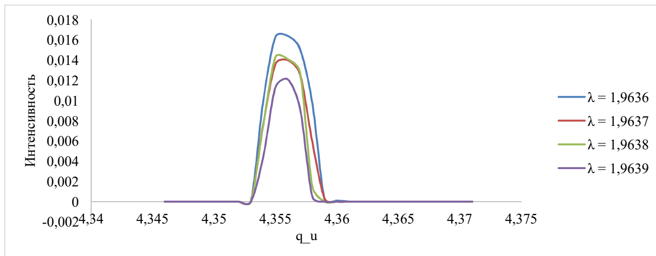
Рис. 1. Влияние углового коэффициента на форму и высоту массовых пиков при работе с одним квадрупольным масс-фильтром
