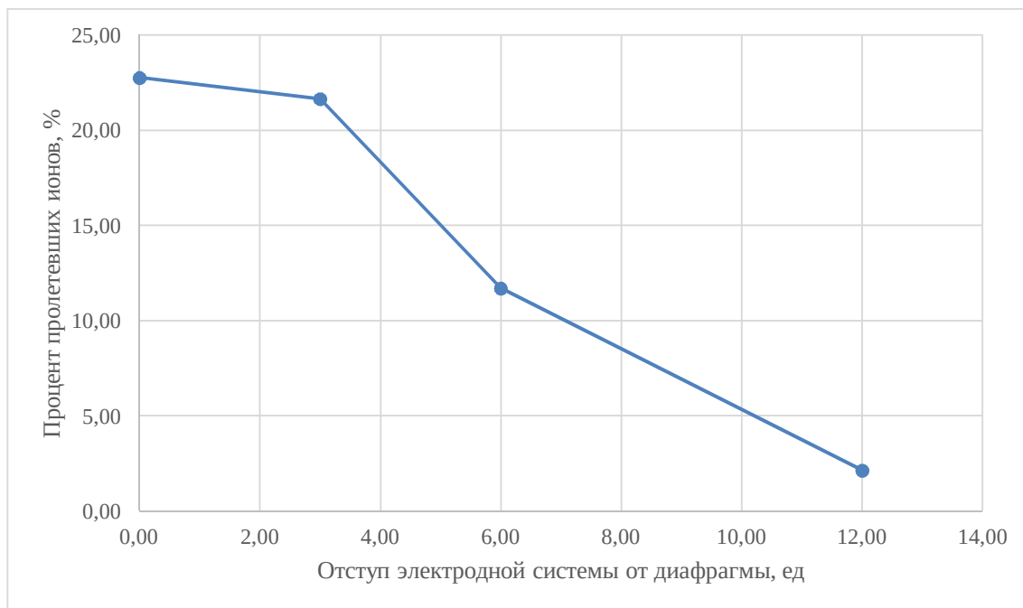
Рис. 2. График зависимости процента пролетевших ионов от величины сдвига электродной системы от входной апертуры
