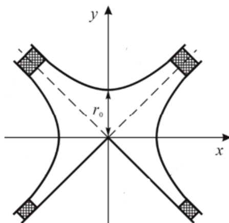
Рис. 1. Конфигурация электродов трипольного анализатора масс с угольным электродом
