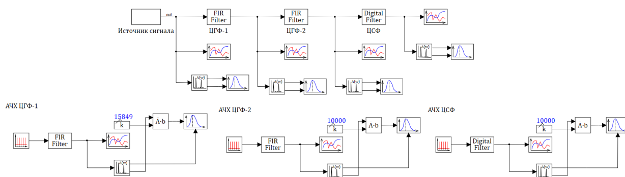
Рис. 4. Модель 3-х ступенчатой гребенчатой структуры КИХ-фильтров
