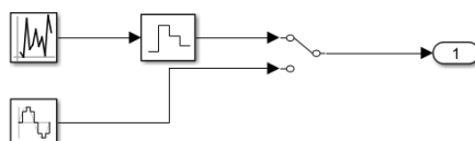
Рис. 3. Подсистема генерации частотного и фазового сдвига
