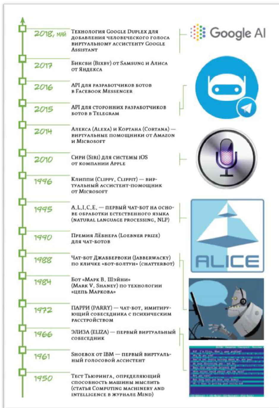
Рис. 3. Эволюция chatbot-технологий
