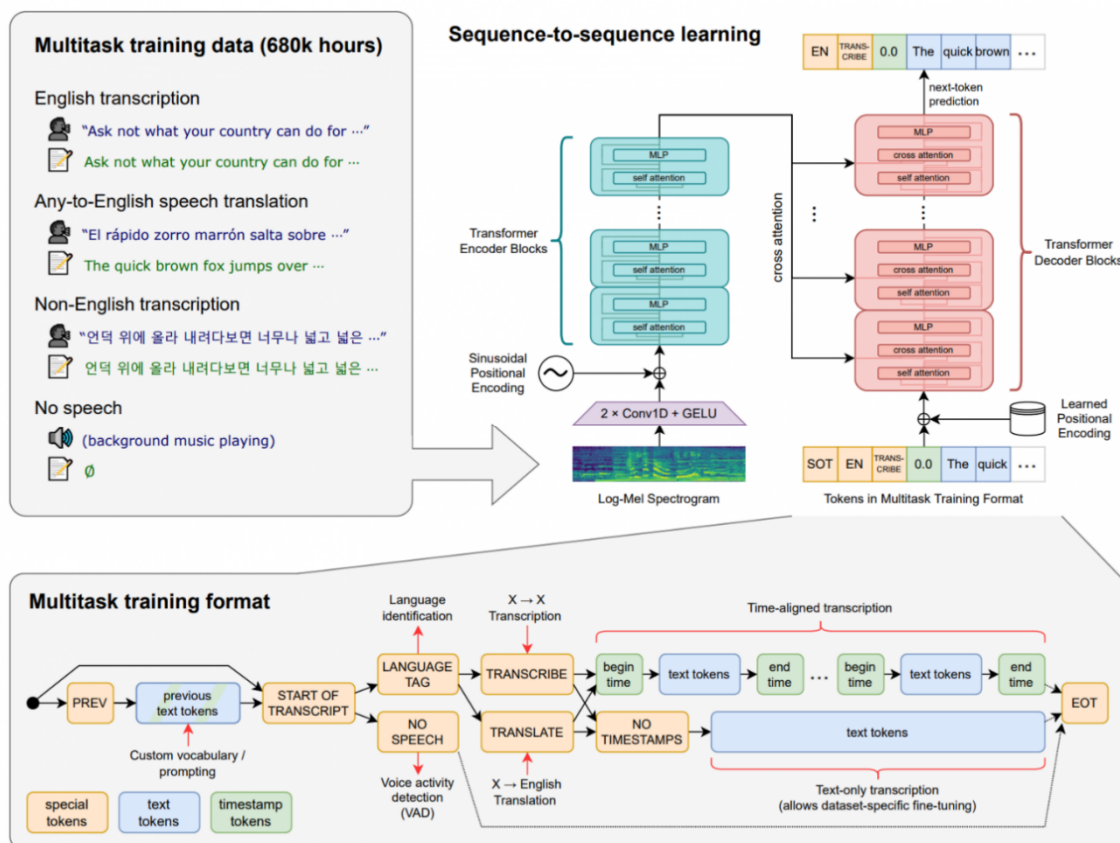
Рис. 9. Архитектура Whisper
