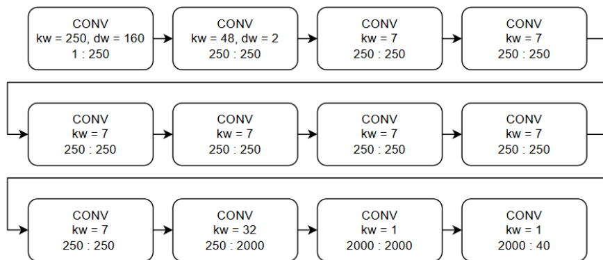
Рис. 5. Архитектура Wav2Letter
