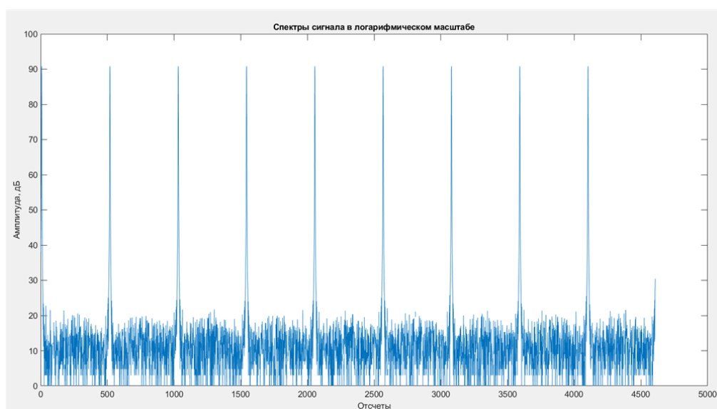
Рис. 2. Результат обработки гармонического сигнала с нулевой доплеровской частотой
