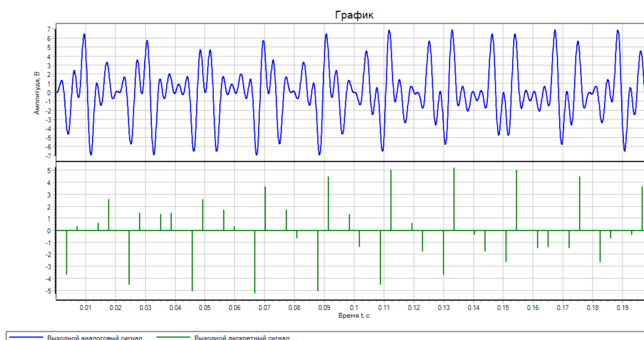
Рис. 5. Выходной аналоговый и дискретный сигналы при частоте дискретизации 285 Гц
