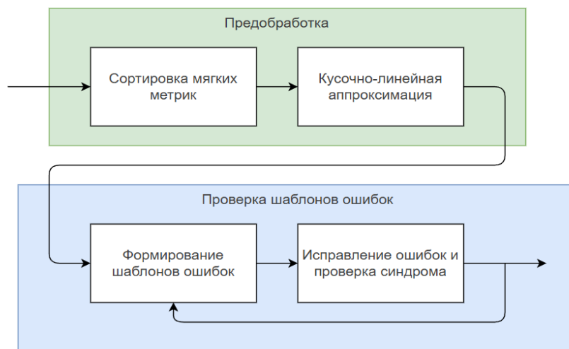
Рис. 2. Структурная схема декодера ORBGRAND
