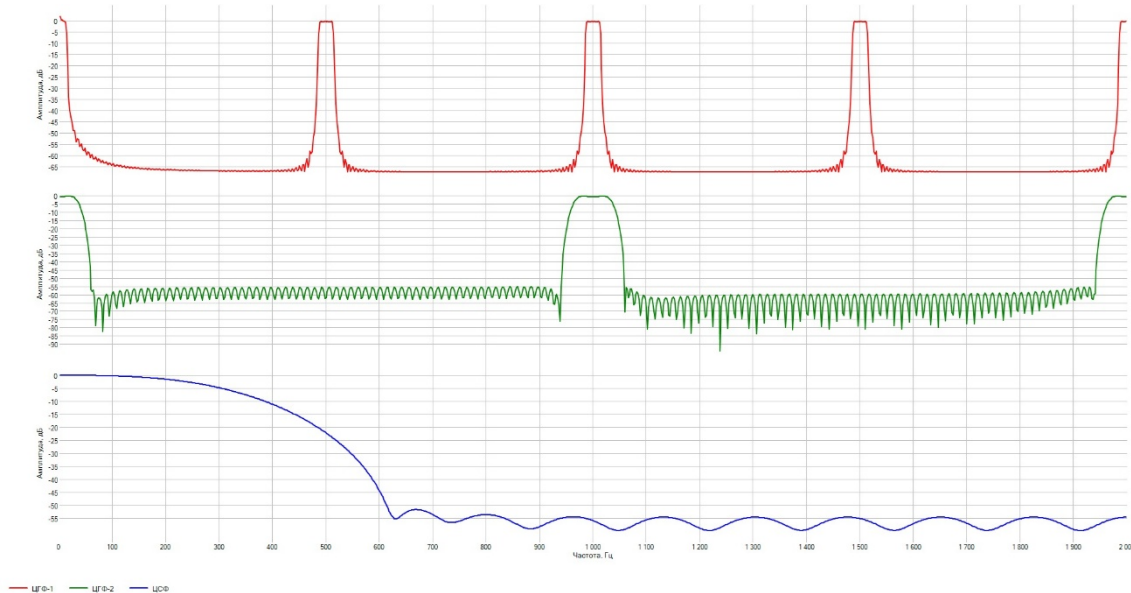
Рис. 5. АЧХ ЦГФ-1 (а), ЦГФ-2 (б) и ЦСФ (в)
