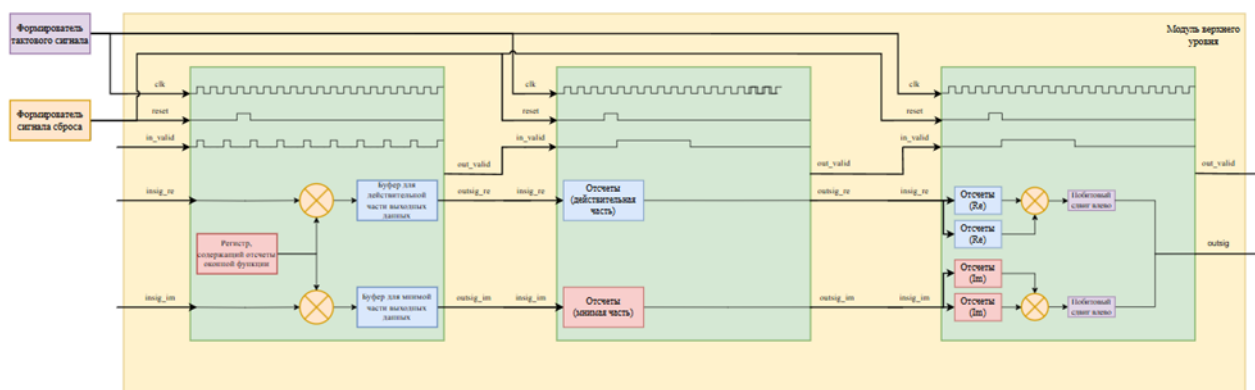
Рис. 1. Структурная схема алгоритма БПФ
