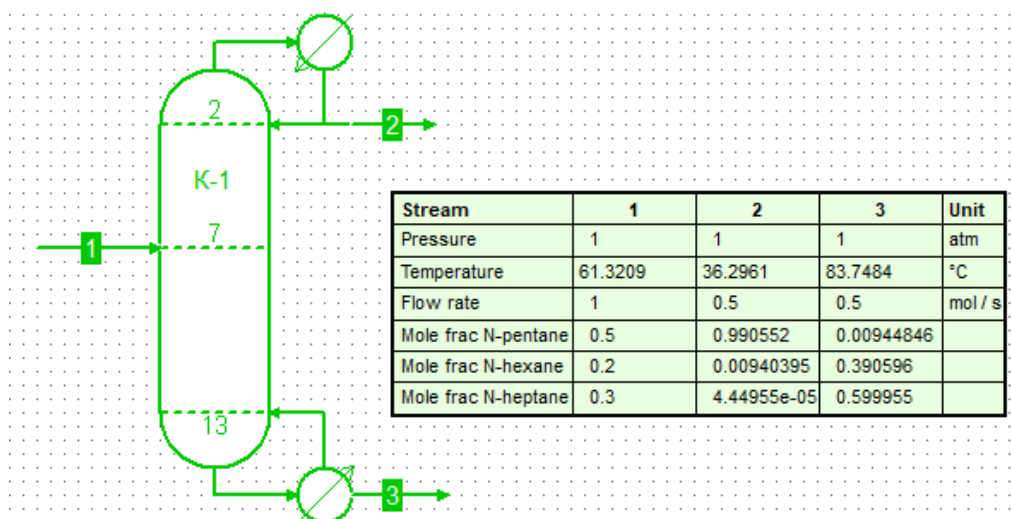
Рис. 4. Рассчитанные программой значение дистиллята
