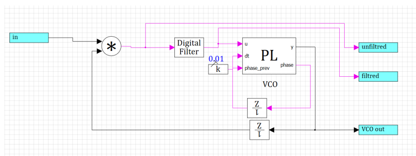
Рис. 9. Подсистема компенсации фазового сдвига
