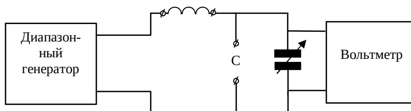
Рис. 2. Структурная схема измерителя добротности
