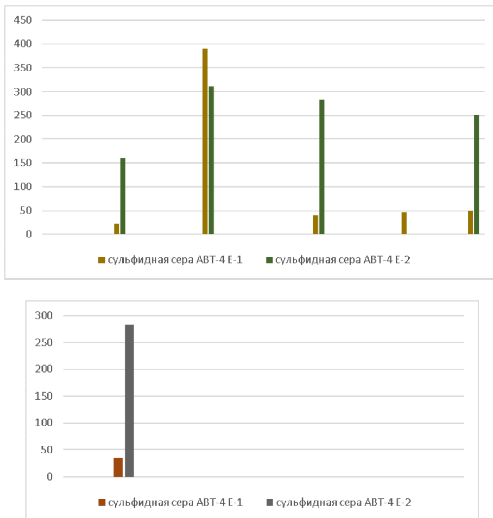
Рис. 4. Результаты измерений S^{2-} дренажной воды из сепаратора бензина Е-1 и Е-2 за 2017 и 2026 год
