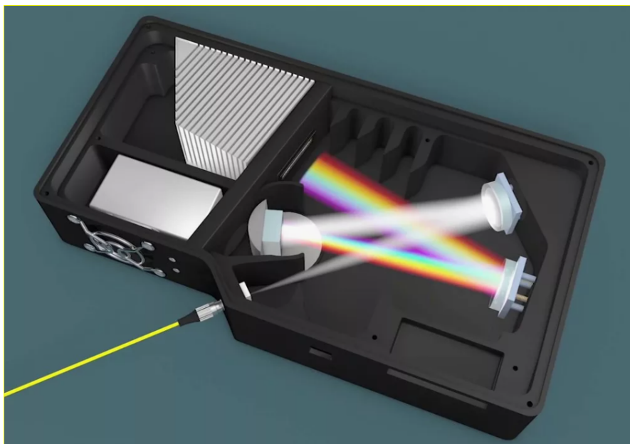
Рис. 1. Портативный дифракционный спектрометр
