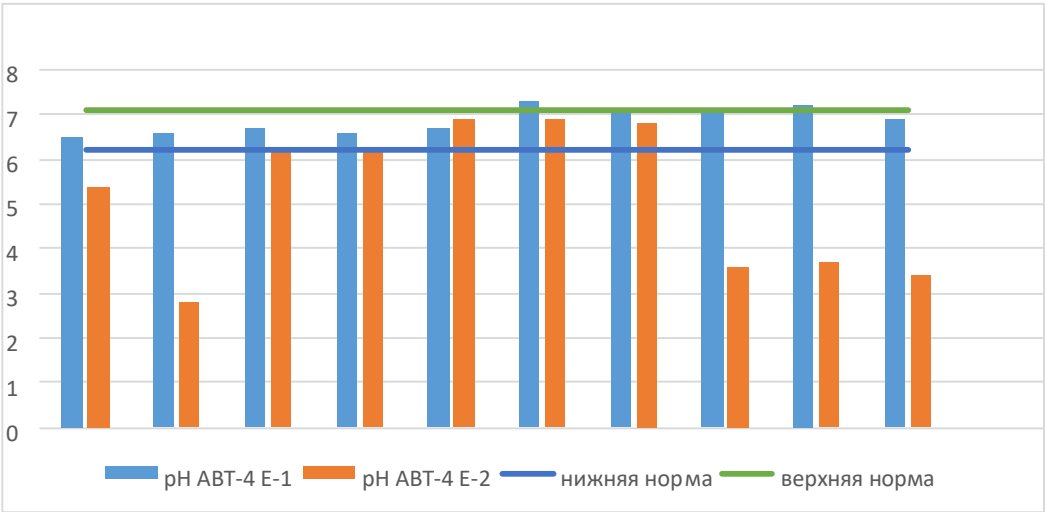
Рис. 1. Результаты измерений pH дренажной воды из сепаратора бензина Е-1 и Е-2 за 2017 и 2026 год Нижняя норма pH- 6,2, верхняя норма pH -7,1
