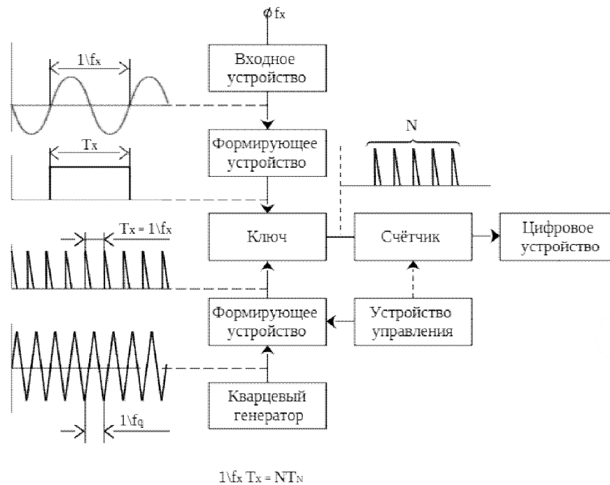
Рис. 3. Структурная схема и временные диаграммы цифрового частотомер, основанного на методе измерения периода
