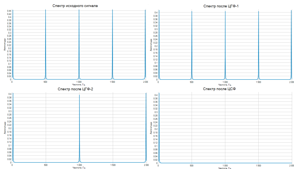
Рис. 6. Спектры исходного сигнала и сигналов на выходах ЦГФ-1, ЦГФ-2 и ЦСФ
