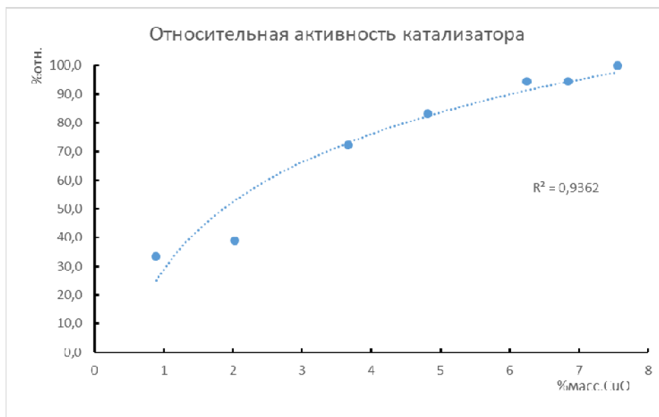
Рис. 2. Показатели относительной активности катализатора в зависимости от концентрации оксида меди
