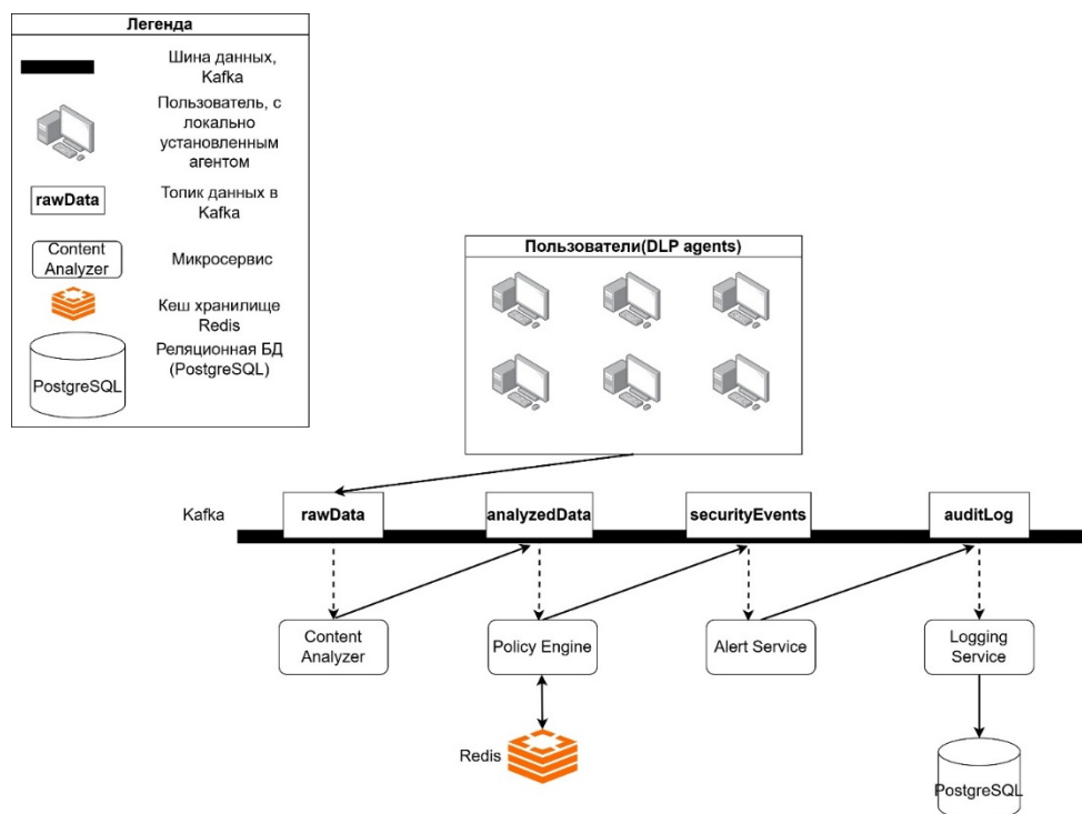
Рис. 1. Схема микросервисной DLP-платформы на базе Apache Kafka
