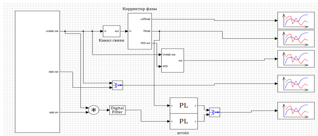
Рис. 7. Схема системы синхронизации в SimInTech
