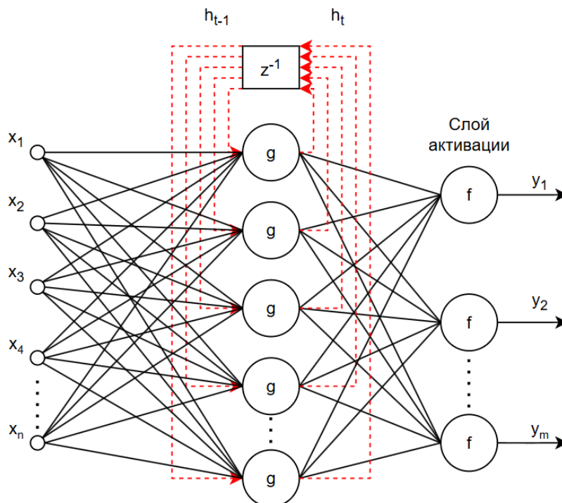
Рис. 1. Рекуррентный слой
