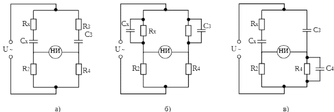
Рис. 1. Схема моста для измерения емкости методом сравнения
