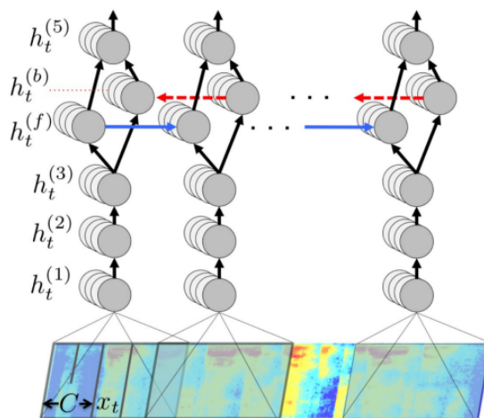
Рис. 5. Структура RNN в Deep Speech
