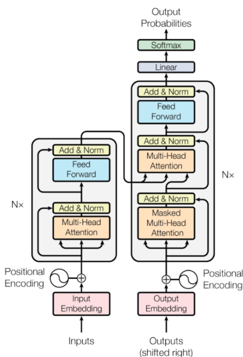
Рис. 7. Архитектура кодер Transformer
