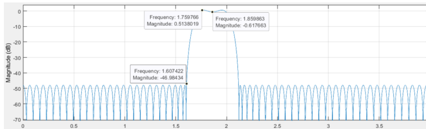
Рис. 2. АЧХ фильтра с порядком 107
