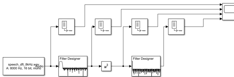
Рис. 3. Детектор огибающей
