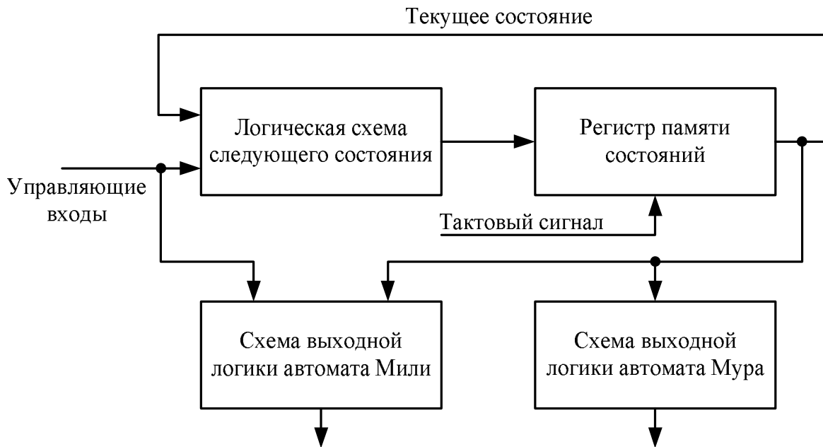
Рис. 1. Структурная схема конечного автомата
