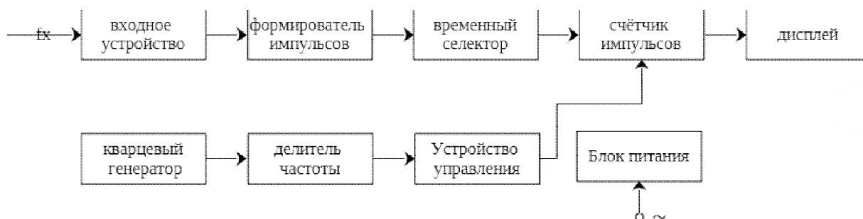
Рис. 2. Структурная схема цифрового частотомера с прямым счётом
