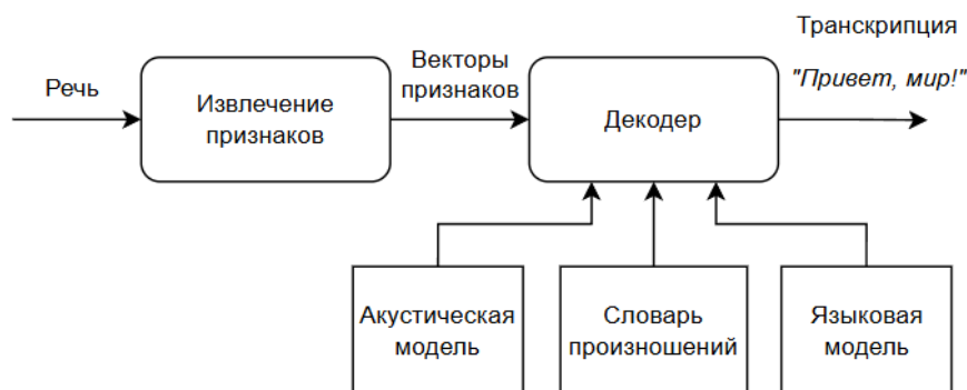
Рис. 4. Архитектура модели на базе НММ
