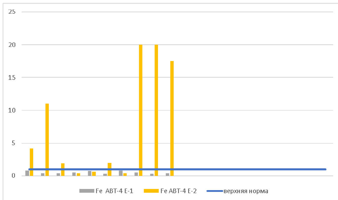
Рис. 2. Результаты измерений \text{Fe}^{3+} дренажной воды из сепаратора бензина Е-1 и Е-2 за 2017 и 2026 год
