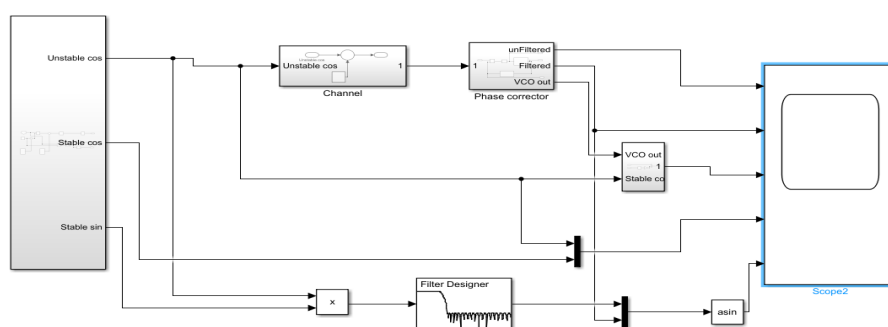
Рис. 1. Схема системы синхронизации в Simulink
