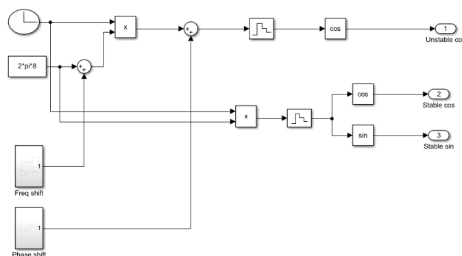
Рис. 2. Подсистема генерации исходного сигнала
