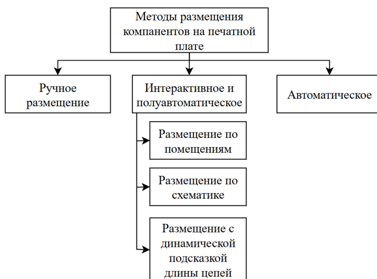
Рис. 1. Классификация методов размещения компонентов на печатной плате
