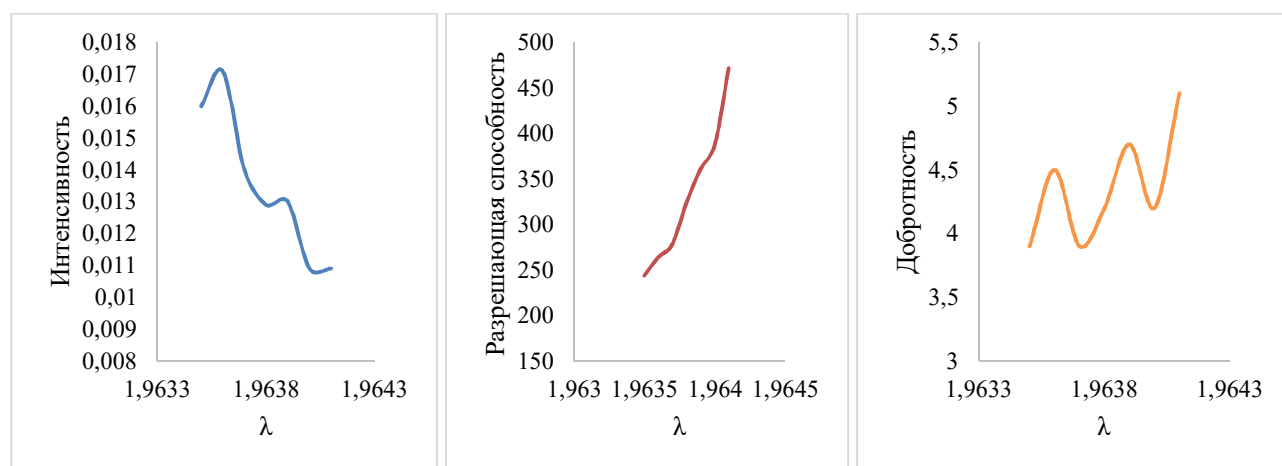
Рис. 4. Зависимости основных качественных характеристик от углового коэффициента при работе с тандемом из двух квадрупольных масс-фильтров
