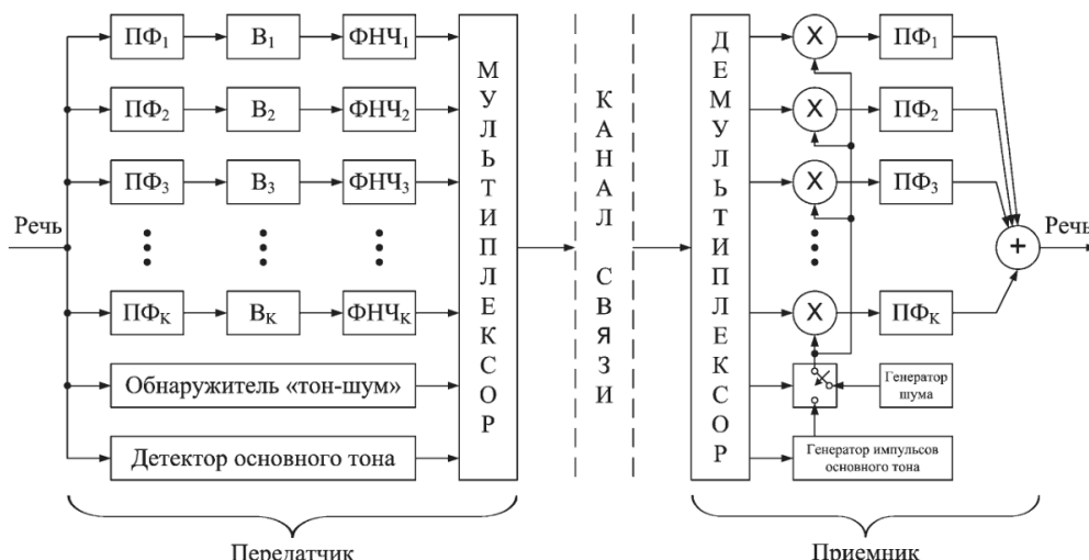
Рис. 1. Структурная схема полосового вокодера
