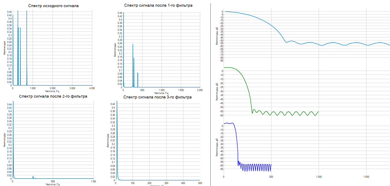
Рис. 3. Спектры исходного сигнала и сигналов на выходе каждого каскада (слева), АЧХ фильтров каждого каскада (справа)
