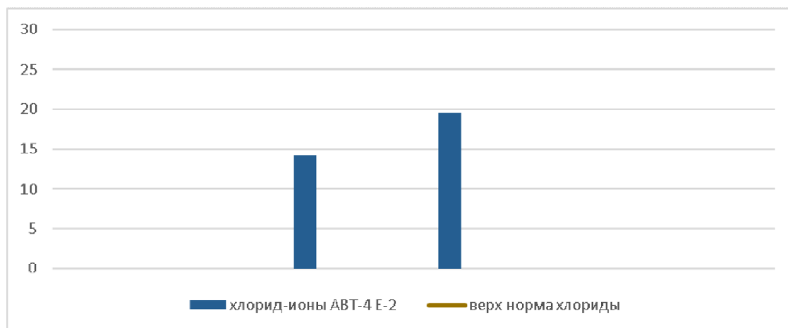
Рис. 3. Результаты измерений \text{Cl}^- дренажной воды из сепаратора бензина Е-1 и Е-2 за 2017 и 2026 год верхняя норма \text{Cl}^- - не более 25 мг/дм³
